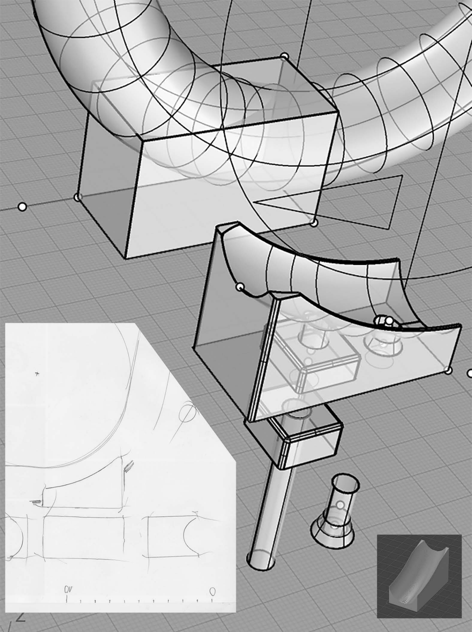
freihandskizze mit drei rissen, masstab (10 cm) für rhino bestimmung des zentrums des fiktiven kreises des rohres
