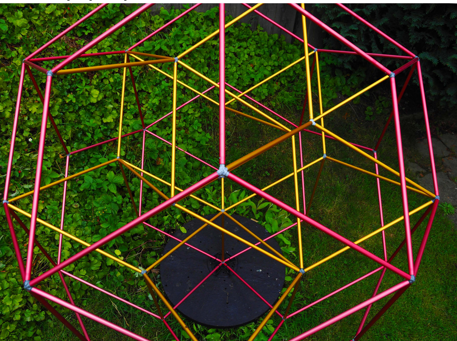
triakontaeder mit einer silberfarbenen diagonalen als visualisierung von einer der sechs dreifachen rotationssymmetrien. keines der drei aluohre hat die genau gleiche länge. 54532 3.6.2026 frs
